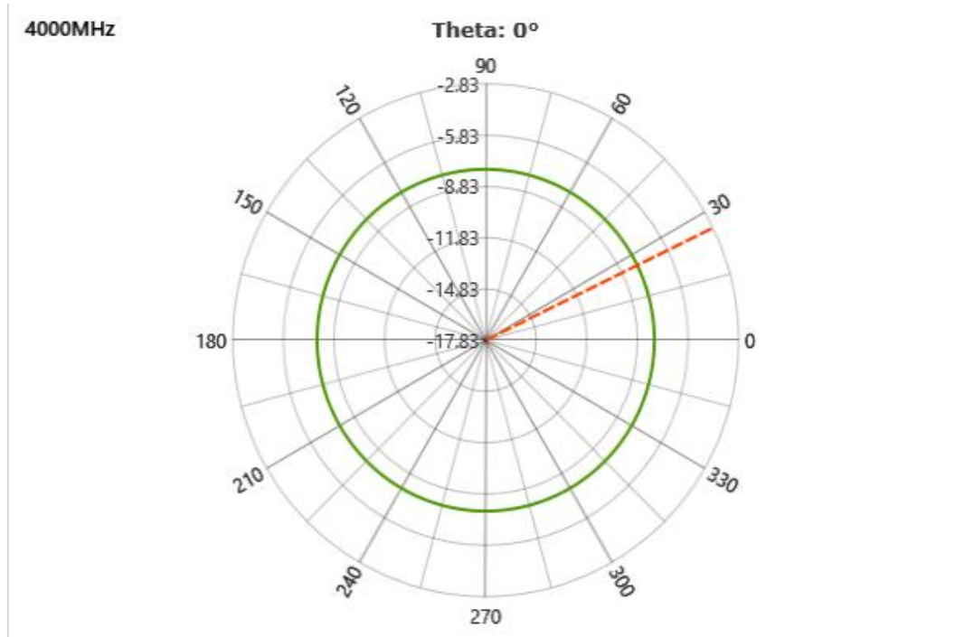
F=4000MHz Horizontal Pattern
