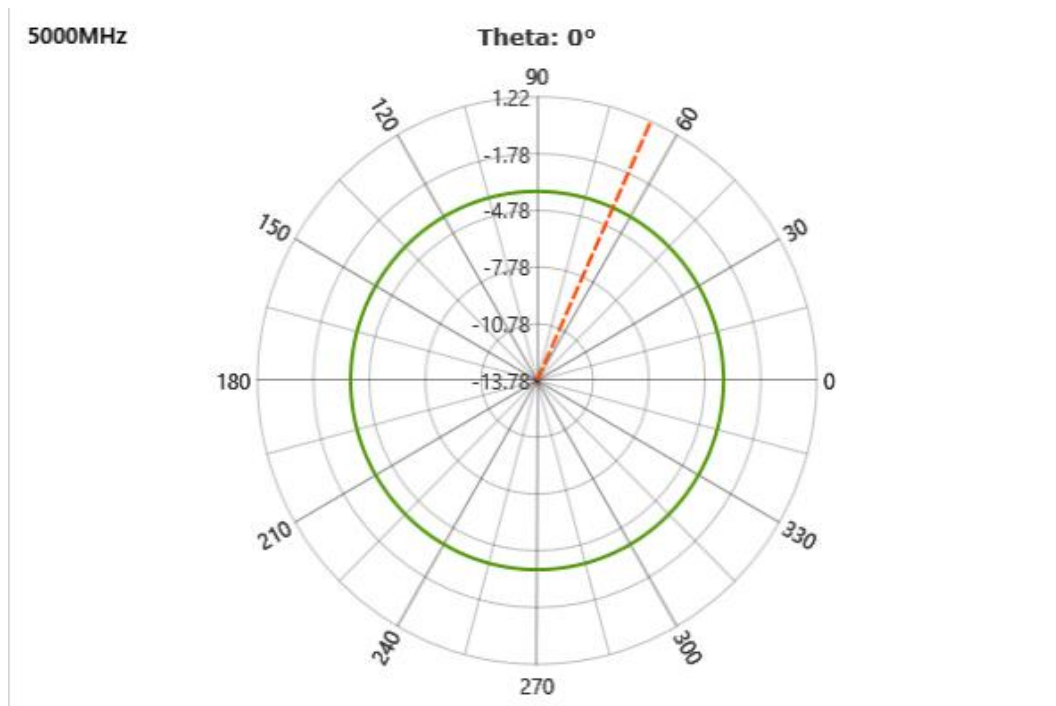
F=5000MHz Horizontal Pattern
